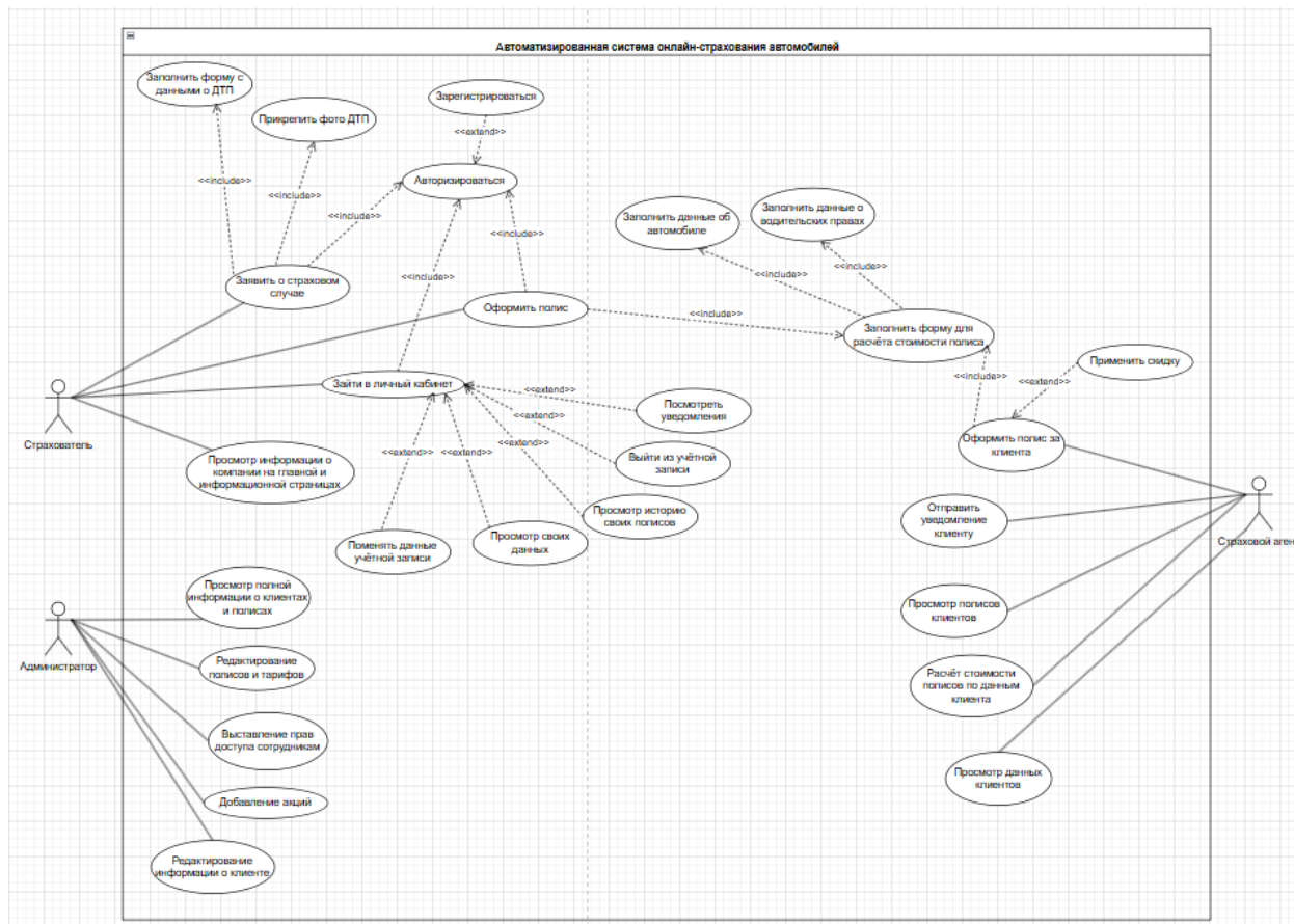
Рисунок 2.5 - UML диаграмма
